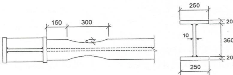
مقطع تیر در خارج از ناحیه کاهش یافته
